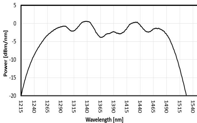
FIG. 1: OSE2 SPECTRUM
