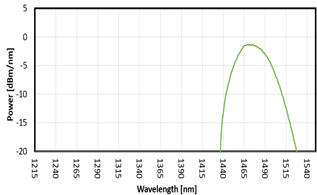
FIG. 2: SLED 1 SPECTRUM
