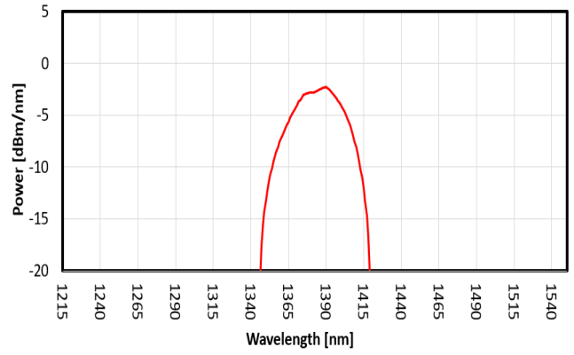
FIG. 4: SLED 3 SPECTRUM
