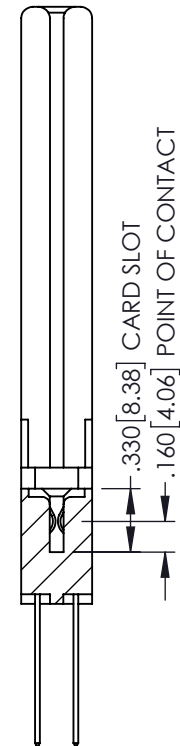
SECTION A-A
