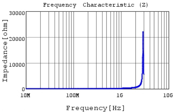
LQG15WH24NJ02 |Z|
