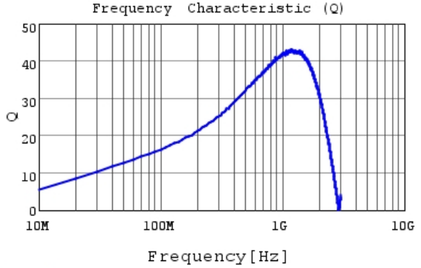
LQG15WH24NJ02 Q
