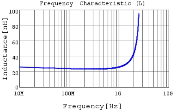
LQG15WH24NJ02 L
