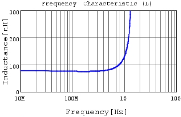
LQG15WH75NH02 L
