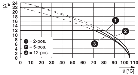
Type: GFKIC 2,5/...-ST-7,62 with GICV 2,5/...-G-7,62
