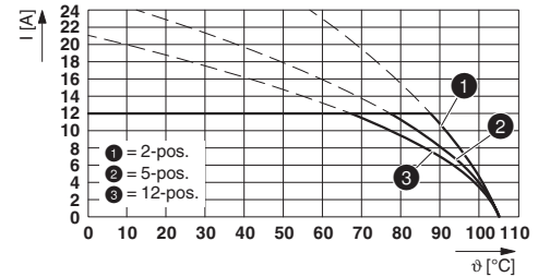
Type: GICV 2,5/...-G-7,62 with GMSTB 2,5/...-G-7,62
