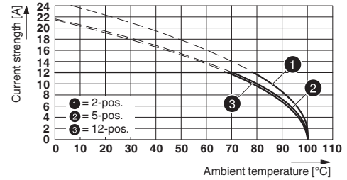
Type: GIC 2,5/...-ST-7,62 with GICV 2,5/...-G-7,62
