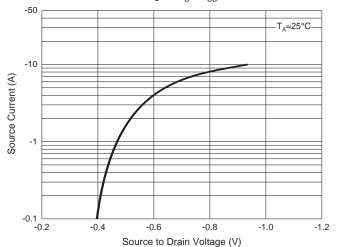
Fig. 6 - I_S — V_{SD}
