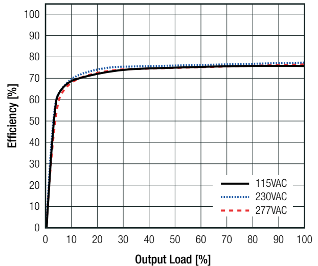
RAC03E-15SK/277
