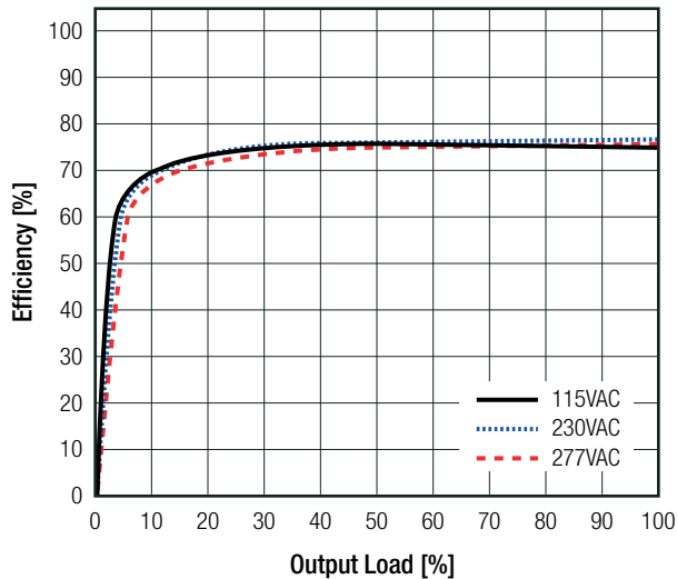
RAC03E-12SK/277 / RAC03E-24SK/277
