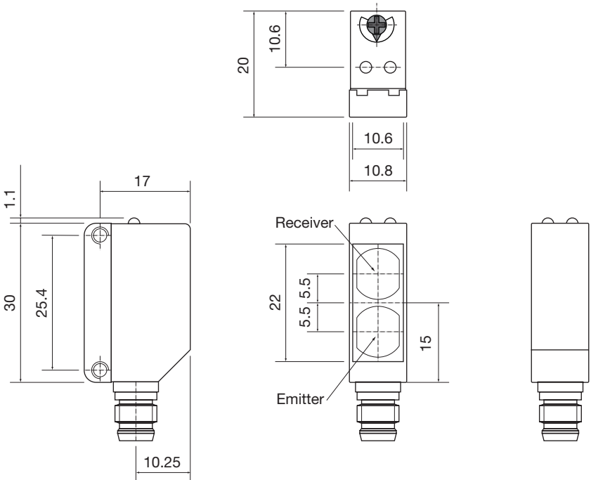
Fig. 6 Plug
