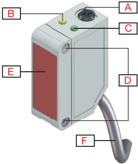
Fig. 1 Cable
