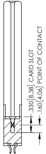
SECTION A-A
