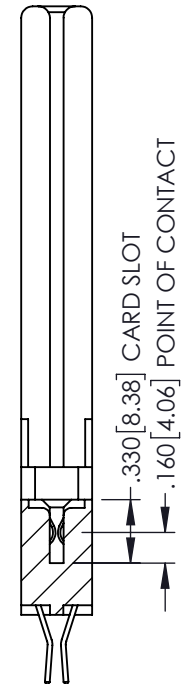
SECTION A-A
