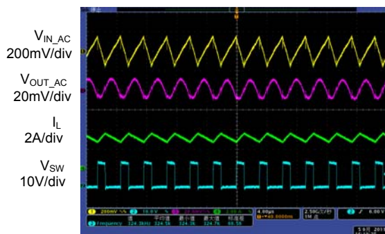
Time 4µs/div
