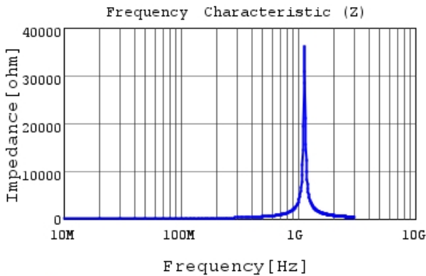
LQG15WHR13J02 |Z|
