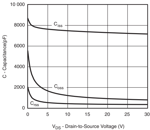
C - Capacitance (pF) C_{iss} C_{oss} C_{rss} V_{DS} - Drain-to-Source Voltage (V) Capacitance
