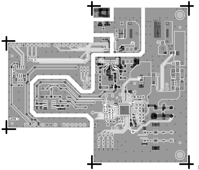
Figure 24. Layer 1, Top Layer
