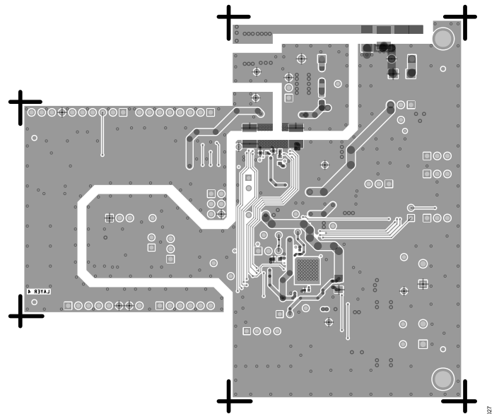
Figure 27. Layer 4, Bottom Layer
