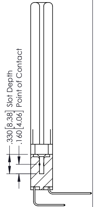
SECTION A-A
