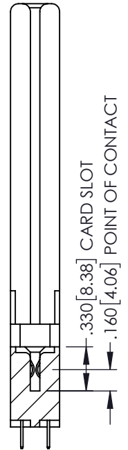
SECTION A-A
