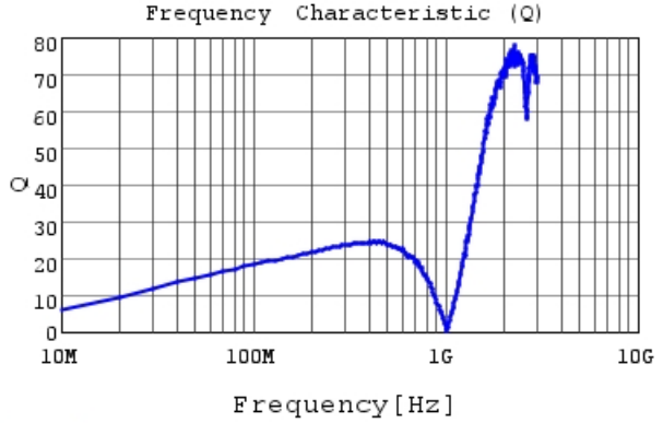
LQG15WHR15H02 Q
