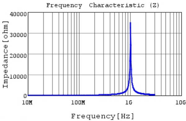
LQG15WHR15H02 |Z|
