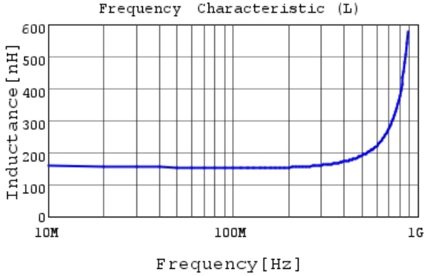
LQG15WHR15H02 L
