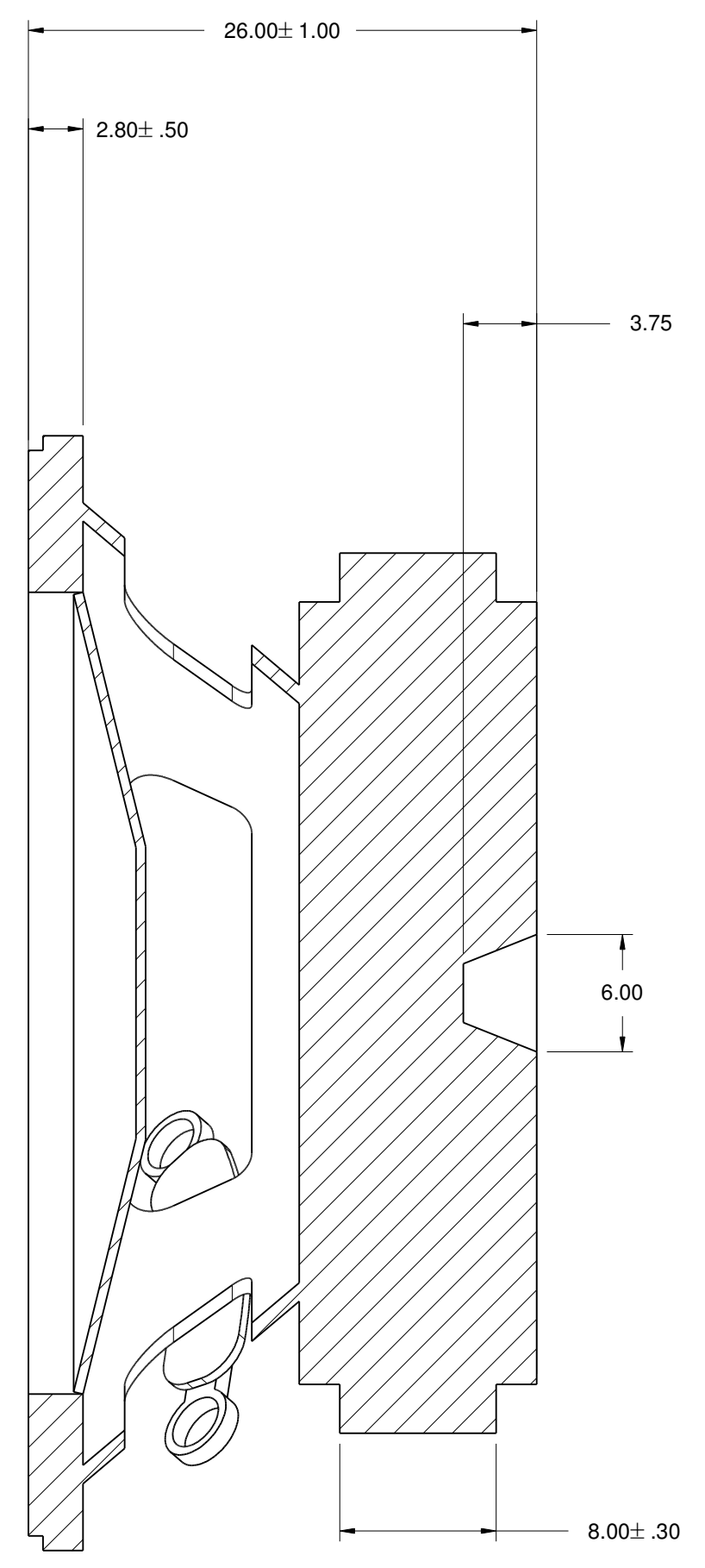
Section A-A
