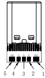
SOLDER PAD POSITION 焊接PIN位示意图
