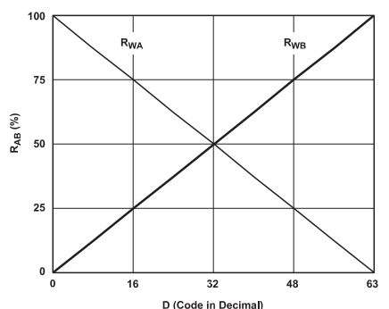
Figure 42. AD5251 R_{WA}(D) and R_{WB}(D) vs. Decimal Code
