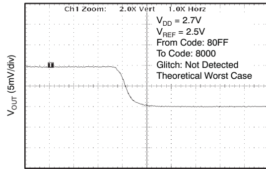
GLITCH ENERGY: 2.7V, 256LSB STEP, FALLING EDGE
