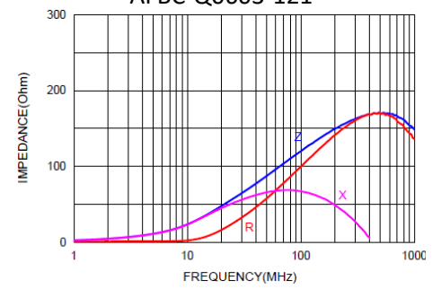
AFBC-Q0603-121
