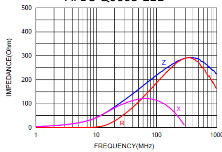
AFBC-Q0603-221
