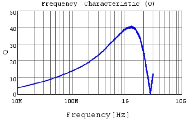
LQG15WH27NJ02 Q
