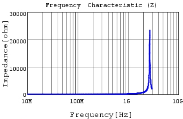
LQG15WH27NJ02 |Z|
