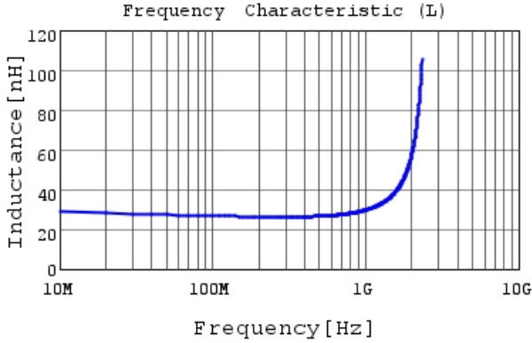
LQG15WH27NJ02 L
