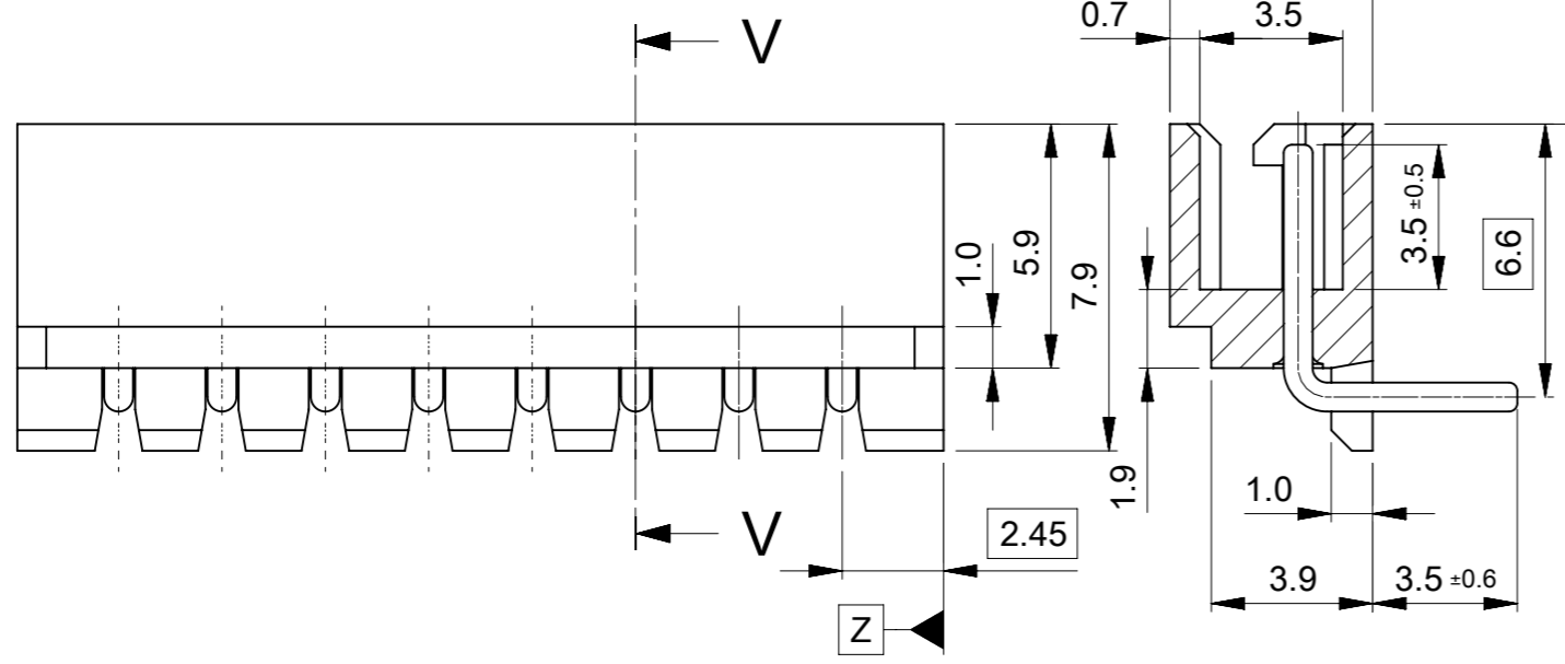
SECTION V-V
