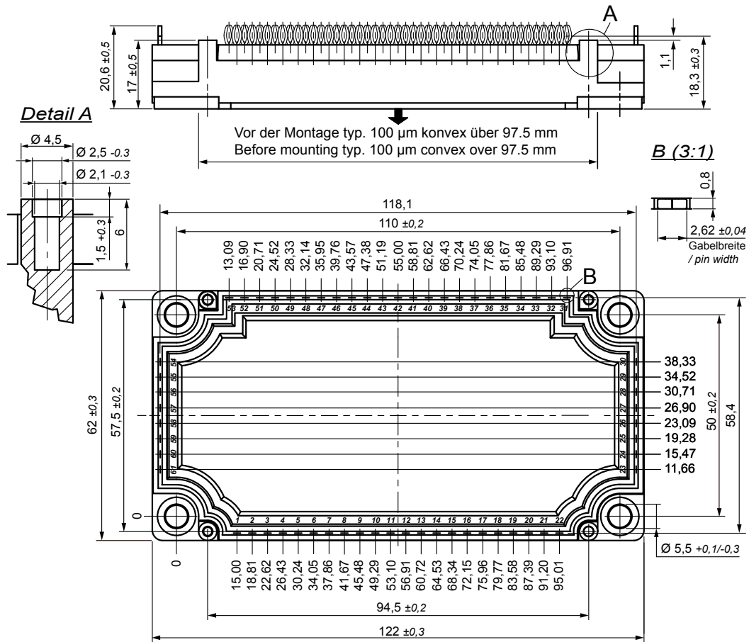
X113a E3-Pack PFP
