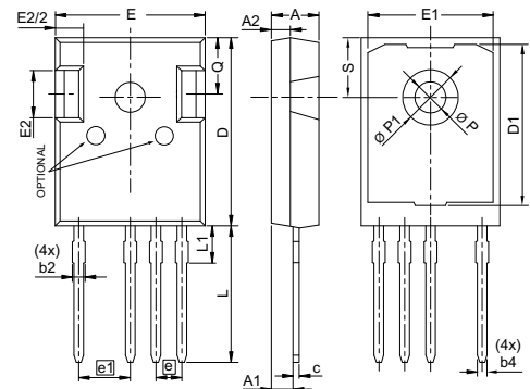
L014d TO-247-4L
