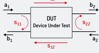
Figure 2: S parameters
