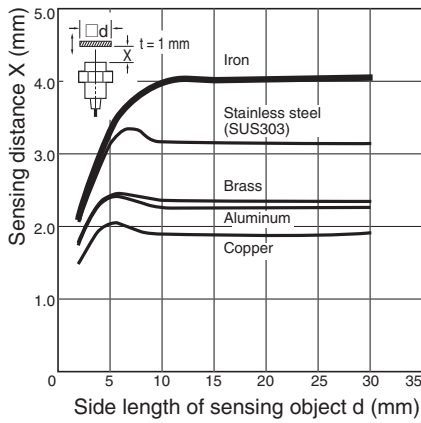
E2AX-M12□S04/ E2A-S12□S04
