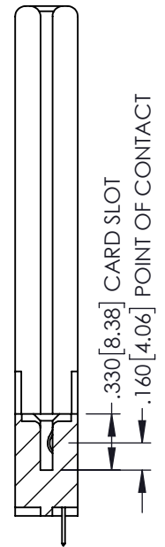
SECTION A-A
