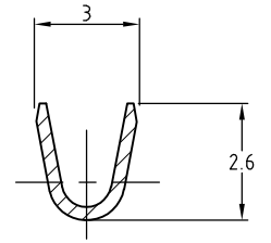
SECT 断面 B-B
