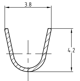
SECT 断面 C-C
