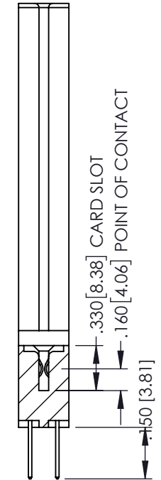
SECTION A-A
