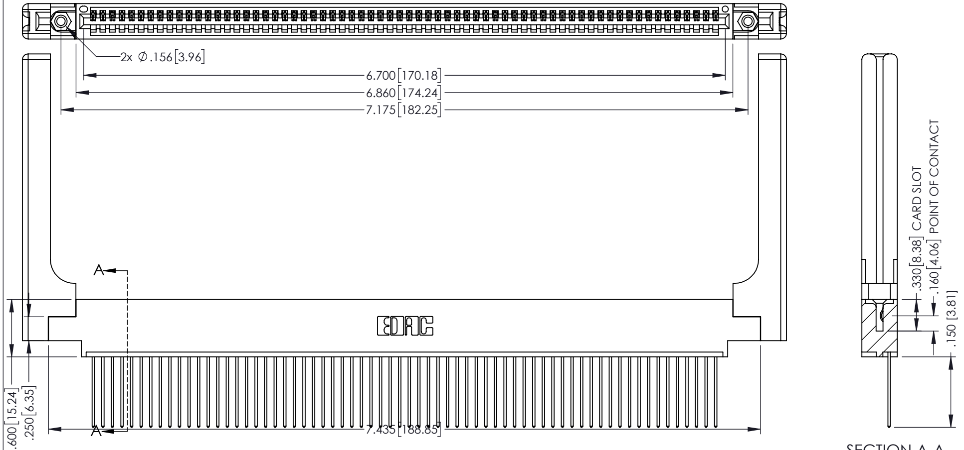
SECTION A-A
