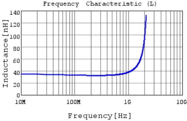
LQG15WH33NH02 L
