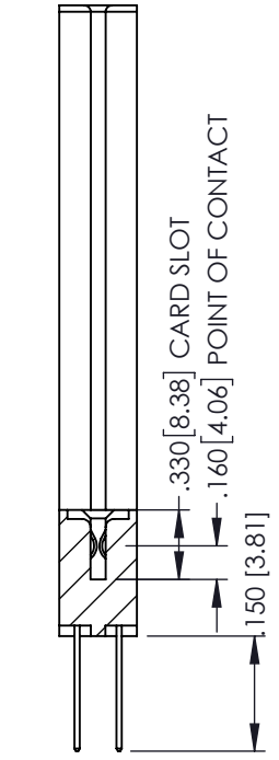
SECTION A-A
