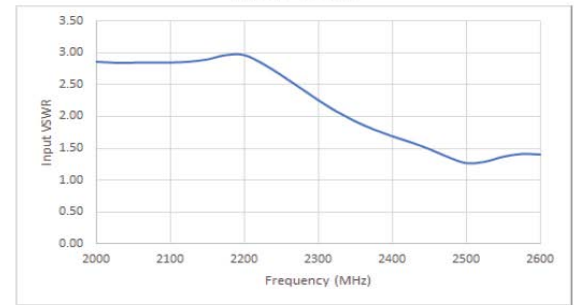
Input VSWR
