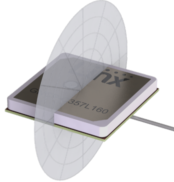
YZ-Plane Gain
