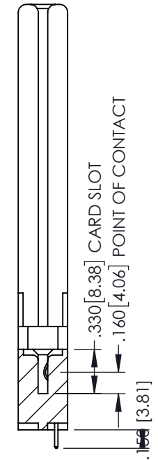
SECTION A-A
