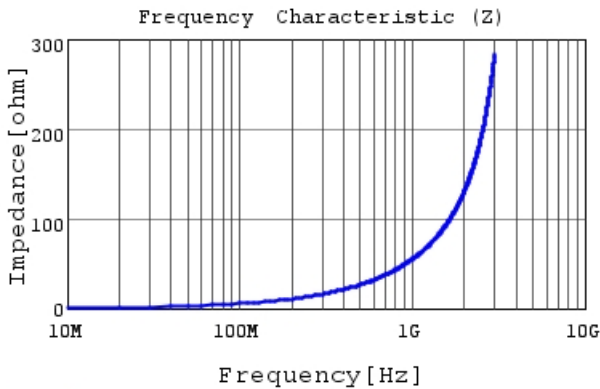
LQG15WH8N7H02 |Z|
