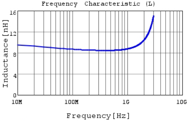
LQG15WH8N7H02 L
