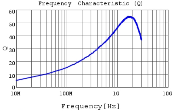
LQG15WH8N7H02 Q
