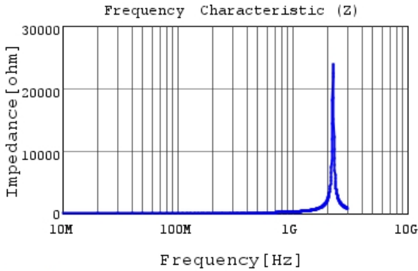
LQG15WH36NJ02 |Z|
