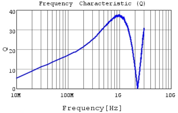
LQG15WH36NJ02 Q
