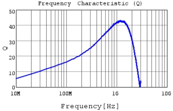
LQG15WZ24NH02 Q
