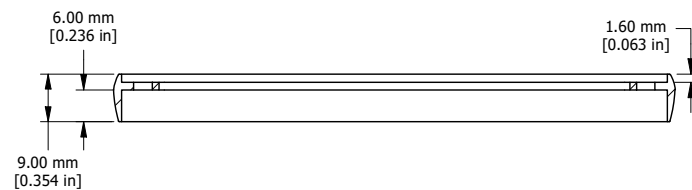
OPEN BEZEL
