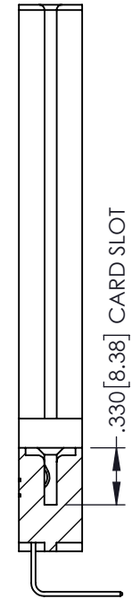
SECTION A-A
