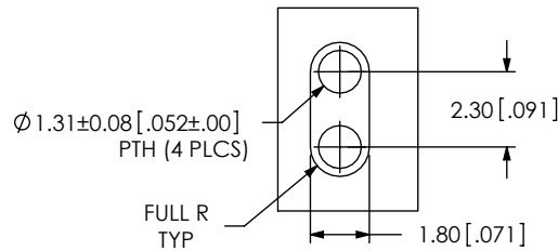
DETAIL 'B' SCALE 4 : 1
