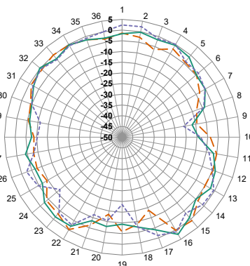
XZ-Plane Gain
