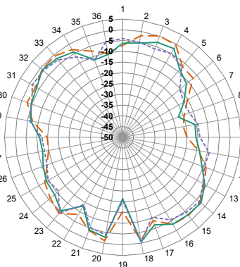
XZ-Plane Gain
