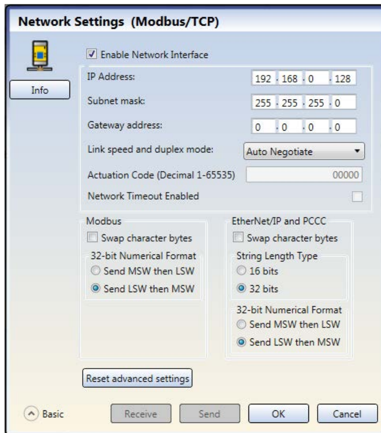
Figure 149. Default Values
