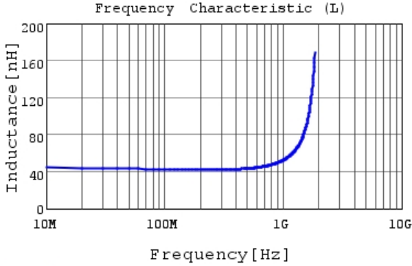
LQG15WZ43NH02 L
