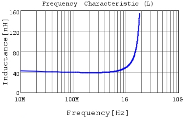
LQG15WH39NG02 L
