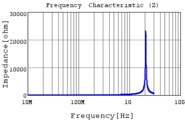
LQG15WH39NG02 |Z|
