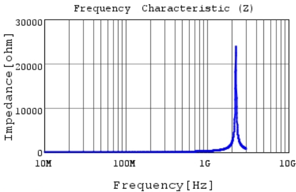
LQG15WZ36NH02 |Z|
