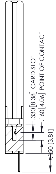
SECTION A-A
