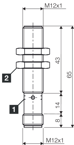
1) LED 4 x 90° (gelb) 2) Schlüsselweite 17 mm BK: schwarz BN: braun BU: blau
