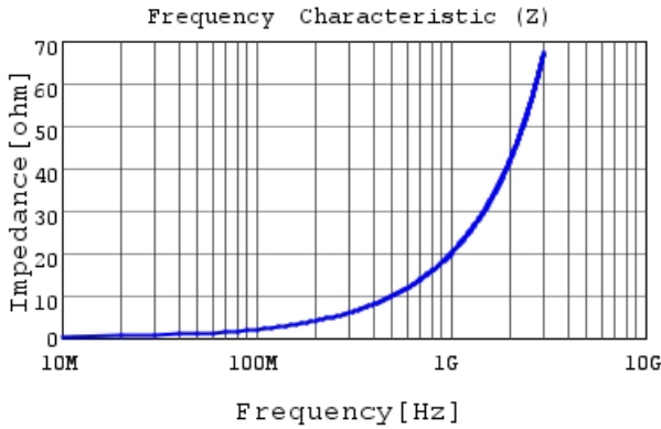
LQG15WH3N2S02 |Z|
